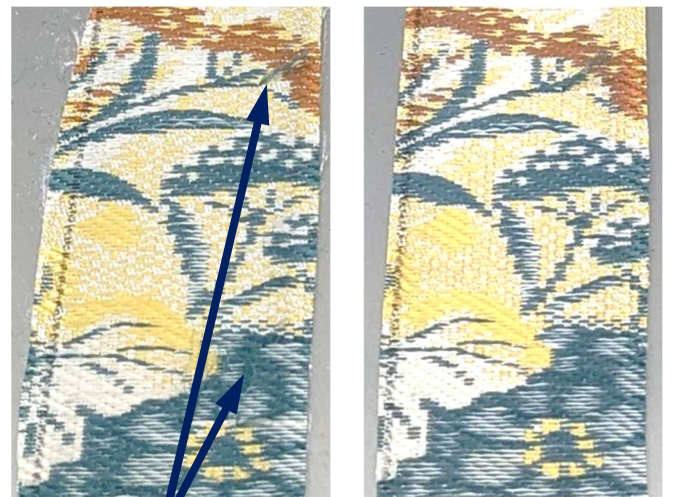
摩擦試験機II形（学振形）による評価
